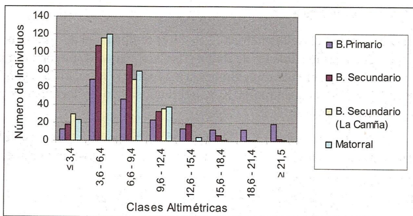
Figura 6. Distribución de los individuos por clases altimétricas en los sitios estudiados, incluyendo individuos con D.A.P \geq 2.5 .
