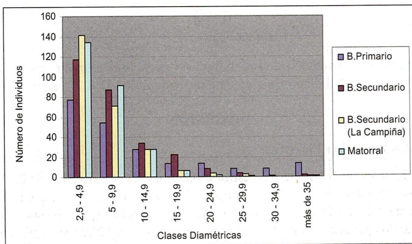
Figura 5. Distribución de los individuos por clases diamétricas en los sitios estudiados, incluyendo individuos con D.A.P \geq 2.5 .
