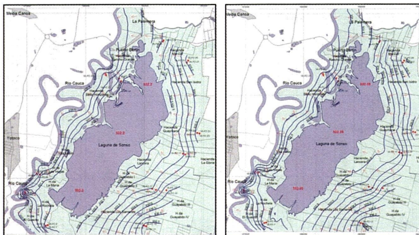
Figura 6. Comportamiento de niveles piezométricos.
