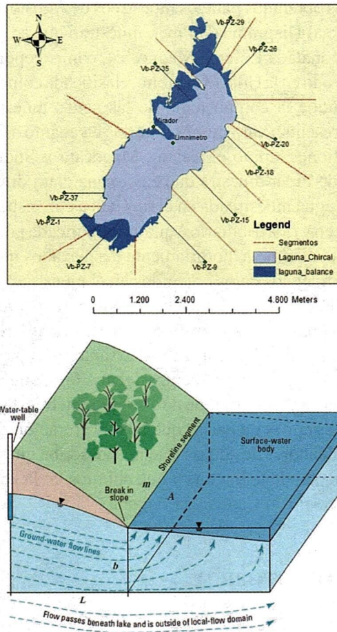
Figura 4. Espaciamiento y distancia de piezómetros a un cuerpo de agua (modificado de Roseberry, 2008).
